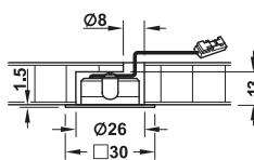
Montaje embutido
