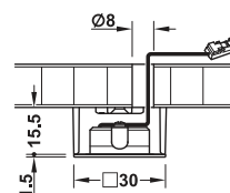
Montaje bajo estantes
