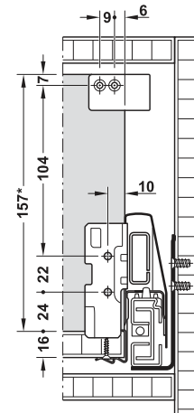
Medidas de montaje panel trasero
