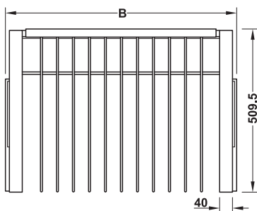
Medidas de montaje
