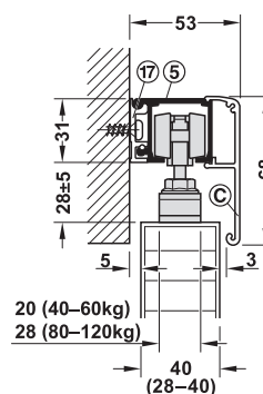
Montaje mural con carril de fijación
