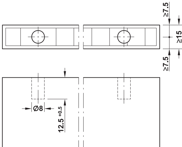
Perforación frontal
