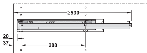
Patrón de perforación
