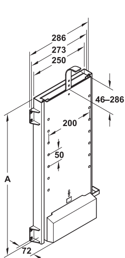
Sistema de elevación
