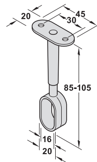
Soporte central/ soporte lateral ajustable en altura
