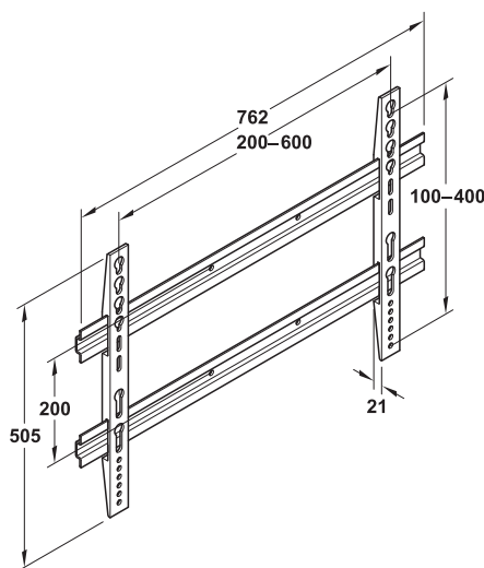
Placa de montaje VESA
