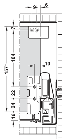
Medidas de montaje panel trasero
