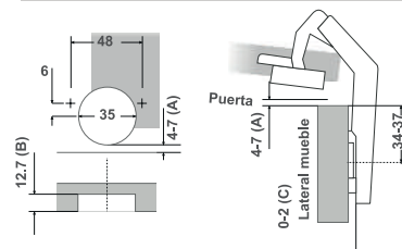
Medidas de la cazoleta para bisagras de 35mm
