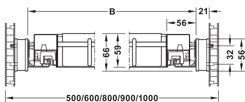
Medidas de montaje
