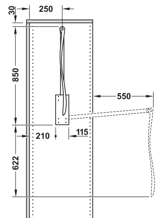
Montaje en el centro del panel lateral del armario
