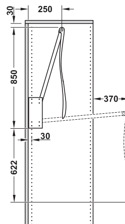
Montaje en el patrón de perforaciones trasero
