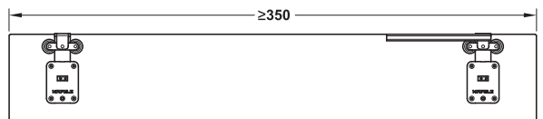
Ancho de puerta mínimo en caso de un amortiguador
