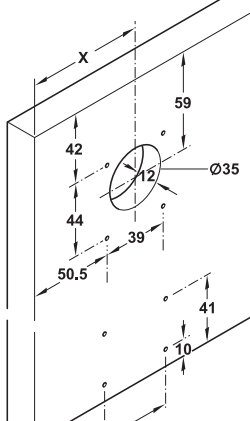
Esquema de taladros
