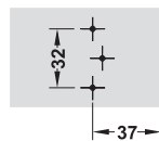
Patrón de perforación
