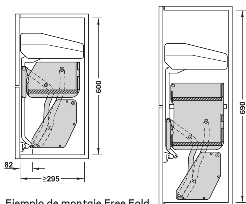
Ejemplo de montaje Free Fold
