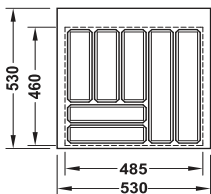
Para ancho de cuerpo 600 mm
