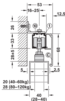
Montaje mural con escuadra de montaje
