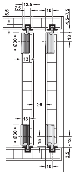
Medidas de montaje
