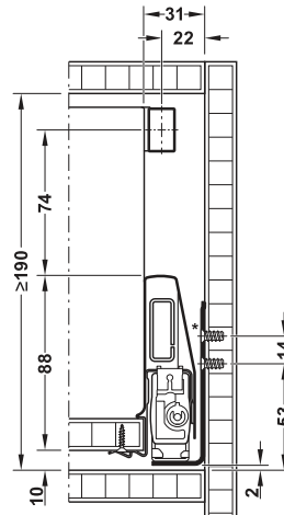
Altura de montaje interior
