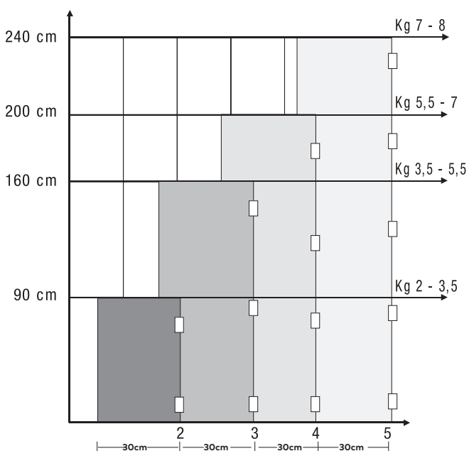
Número de bisagras de cazoleta por puerta según su tamaño y peso:
