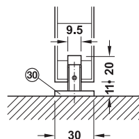
Guía de suelo sin holgura sin carril guía
