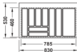
Para ancho de cuerpo 900 mm
